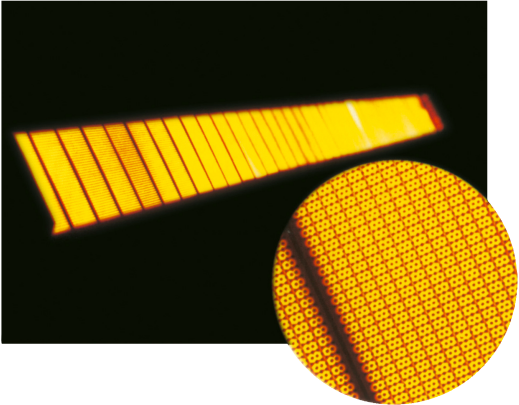
Quemador cerámico de gas sin necesidad de mantenimiento para minimizar los tiempos de inactividad. 20% más eficiente que los quemadores de llama azul normales. Un quemador único y patentado por Electrolux Profesional.
